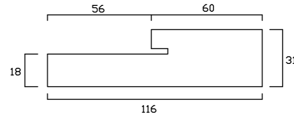
上枠・縦枠
